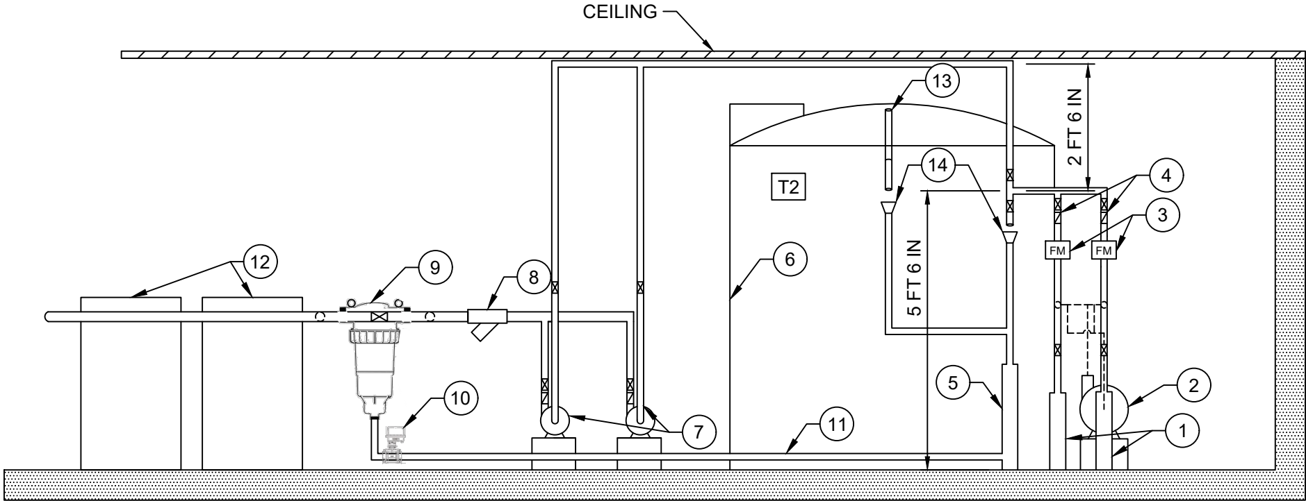
A SECTION A-A'
